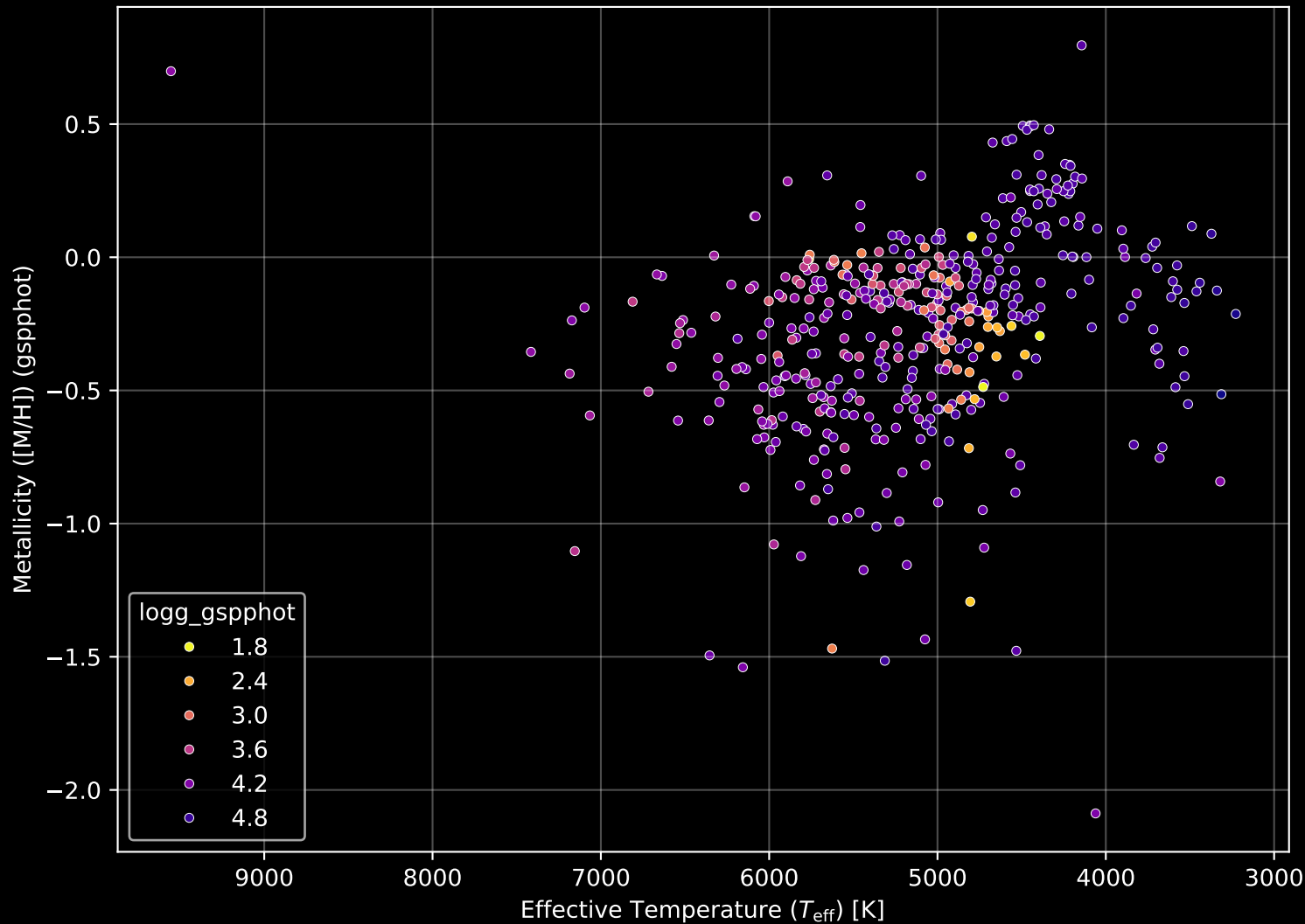
APOGEE DR17 Field: [GD1-3] Stellar Population Parameters (n= 448)
